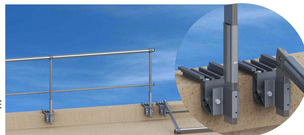
GARDE-CORPS SABOT Z RABATTABLE RÉF. : VZ-R1 / VZ-R2 / VZ60-R1 / VZ60-R2 VZ100-R1 / VZ100-R2 / VZ140-R1 / VZ140-R2
