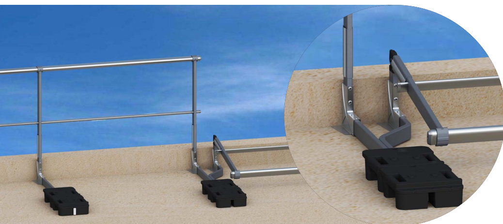
GARDE-CORPS AUTOPORTANT RABATTABLE RÉF. : VAP-R2 / VAP-R3
